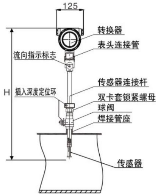
插入式外形
