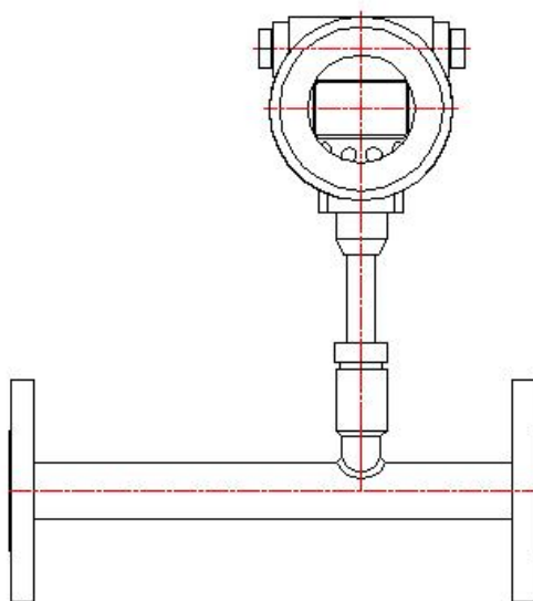
插入式外形
